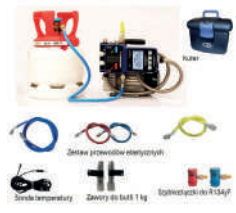
Zestaw do obsługi klimatyzacji IdeaTronics CS
